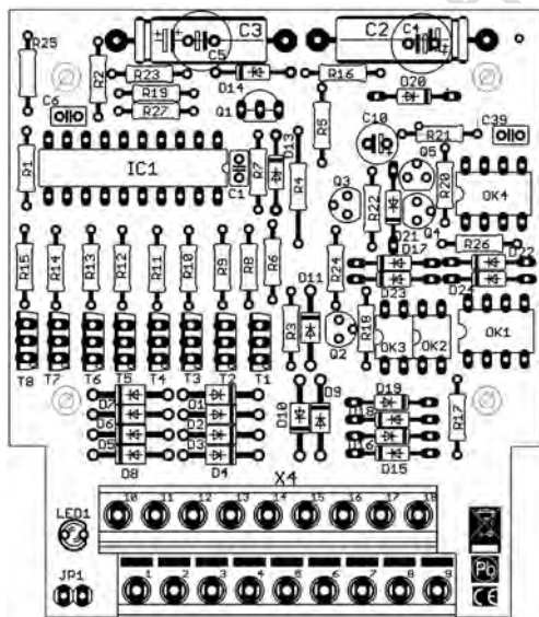
Fig. 1: Bestückungsplan (WD-34)
